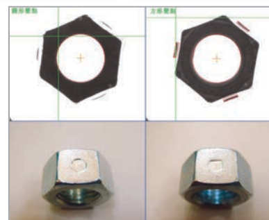
360° 外部檢測 360° External Inspection
